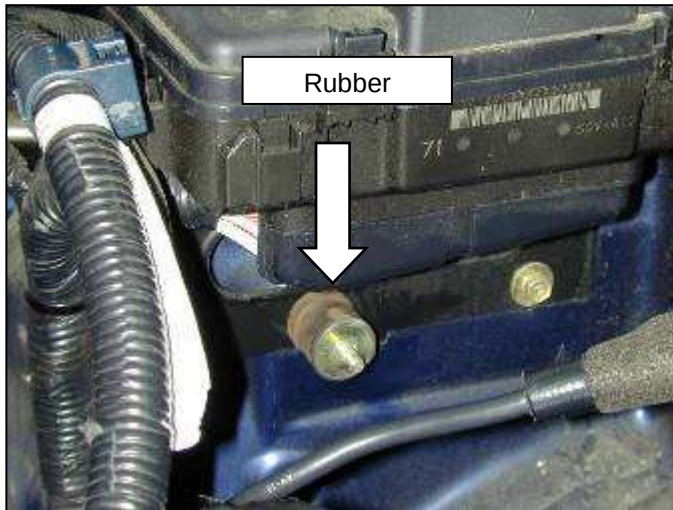
b. Install 6mm rubber mount.
